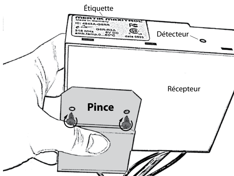
Fixation de la pince au récepteur
