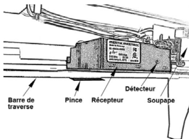
Récepteur en position finale sur la traverse de fonte
