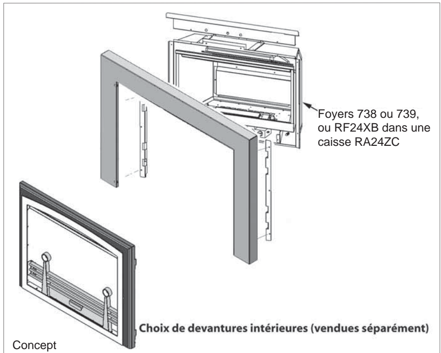
Bordure angulaire 756 montrée avec la Porte simple FenderFire 744FV1 optionnelle (D'autres devantures sont disponibles)
