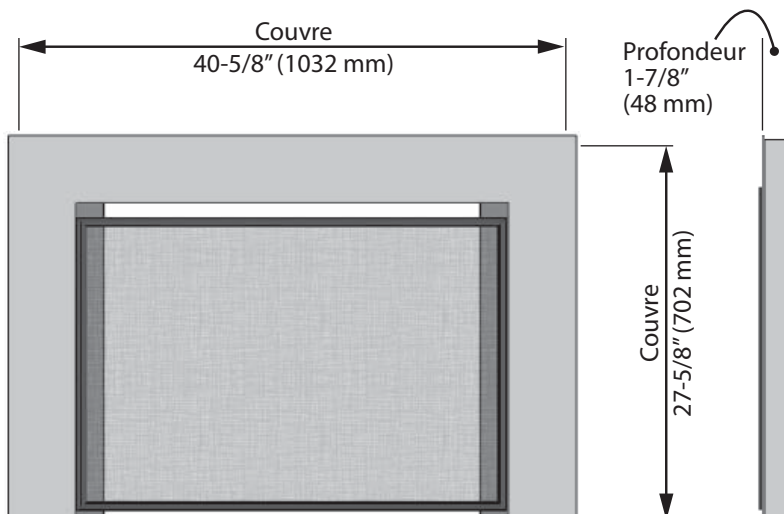
Façade de la bordure légèrement plus grande
